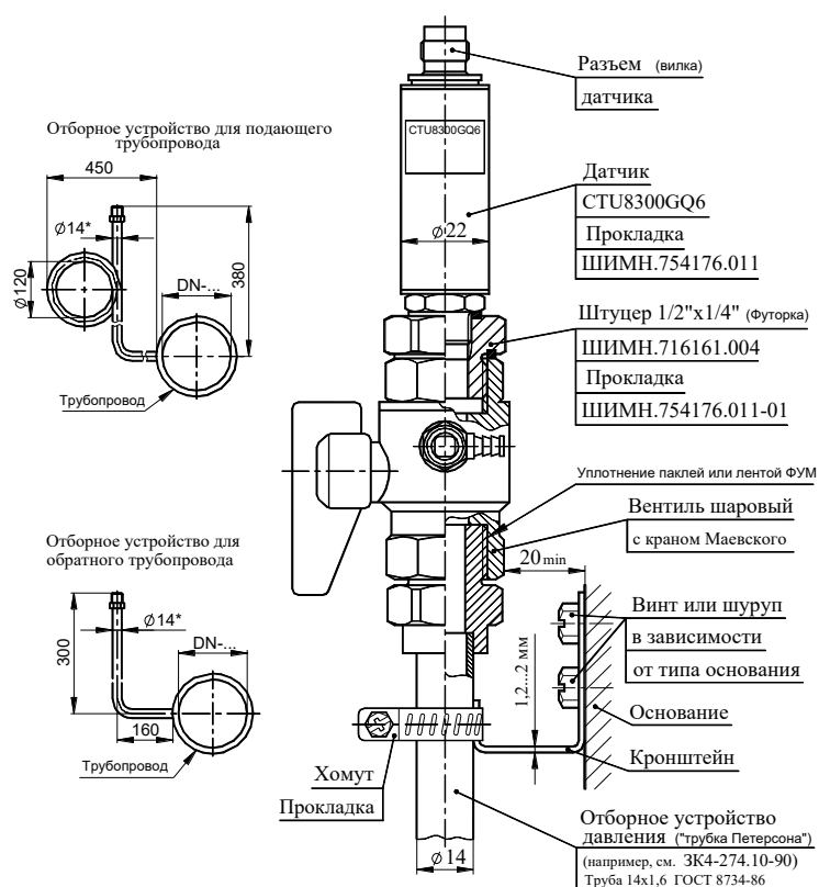
Рис. 5. Рекомендована схема встановлення датчика тиску (на прикладі датчика STU8300GQ6) і розміри добірних пристроїв тиску
