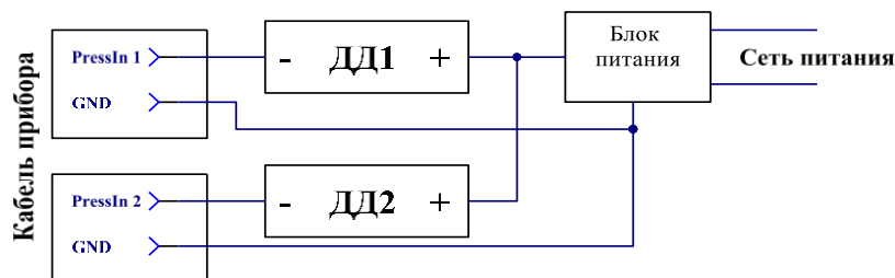
Рис. 8. Підключення ДД при використанні зовнішнього блоку живлення.
