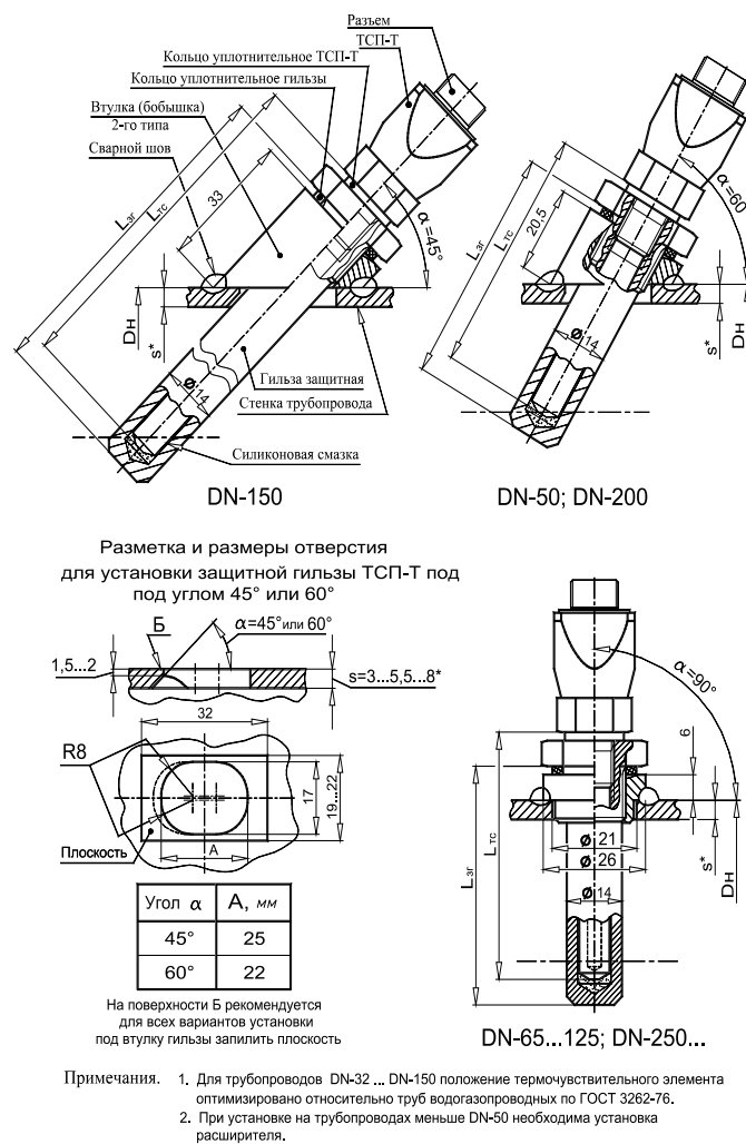
Рис. 4. Встановлення ТСП-Т типів 2, 3, 4 з захисної гільзою
