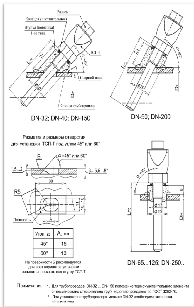
Рис. 3. Встановлення ТСП-Т типів 2, 3, 4 без захисної гільзи
