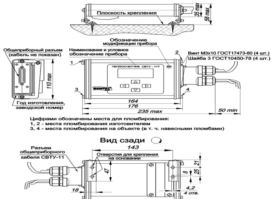
Рис.6. Обчислювач: зовнішній вигляд, габаритні розміри.
